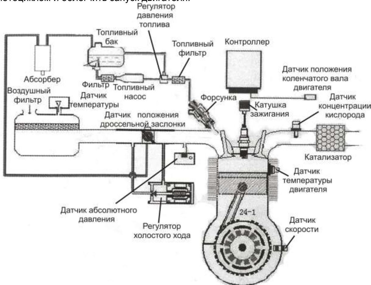
Рис. 16. Схема системы впрыска
